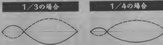
▼図2 節によって生じる振動例
