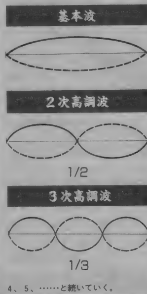
▼図1 弦振動の倍音
